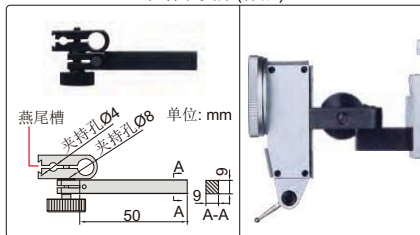
杠杆表支架(标配)
