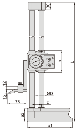
单位: mm
